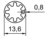
PROFİL NO : 250 AĞIRLIK : 0.171 Kg/m
