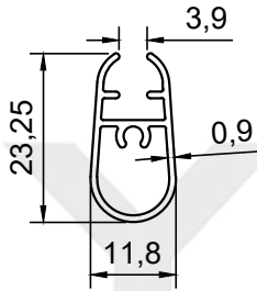
PROFİL NO : 251 AĞIRLIK : 0.179 Kg/m
