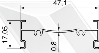
PROFİL NO : 253 AĞIRLIK : 0.241 Kg/m
