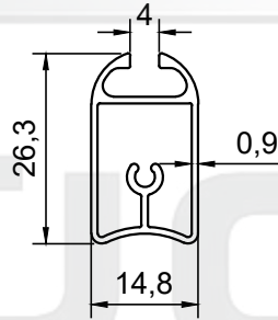
PROFİL NO : 256 AĞIRLIK : 0.255 Kg/m
