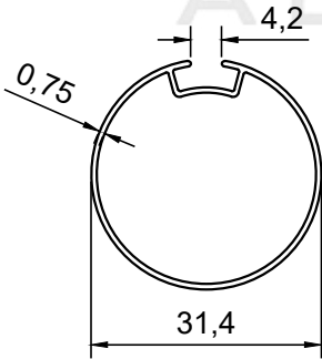
PROFİL NO : 258 AĞIRLIK : 0.214 Kg/m
