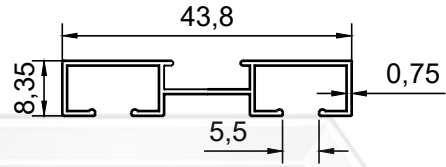
PROFİL NO : 1677 AĞIRLIK : 0.192 Kg/m
