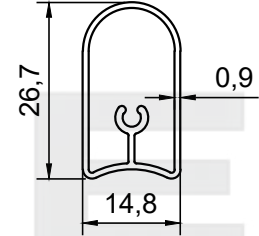
PROFİL NO : 257 AĞIRLIK : 0.220 Kg/m
