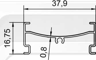
PROFİL NO : 254 AĞIRLIK : 0.198 Kg/m
