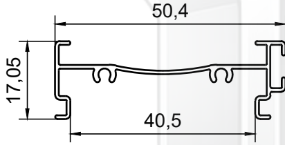
PROFİL NO : 255 AĞIRLIK : 0.265 Kg/m
