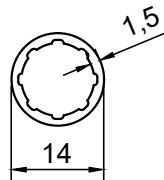
PROFİL NO : 252 AĞIRLIK : 0.144 Kg/m
