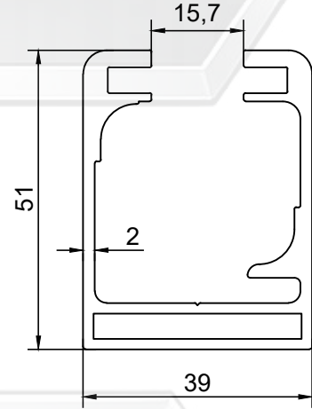
PROFİL NO : 134 AĞIRLIK : 1.315 Kg/m
