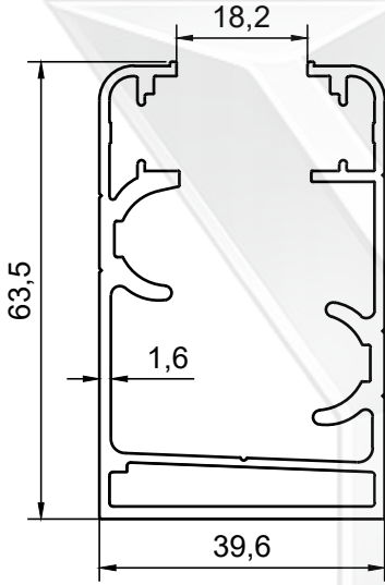
PROFİL NO : 2056 AĞIRLIK : 1.244 Kg/m
