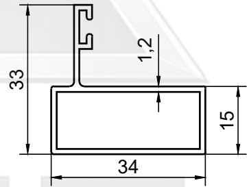
PROFİL NO : 135 AĞIRLIK : 0.393 Kg/m
