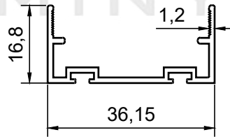
PROFİL NO : 1503 AĞIRLIK : 0.266 Kg/m
