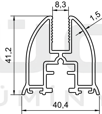
PROFİL NO : 322 AĞIRLIK : 0.932 Kg/m
