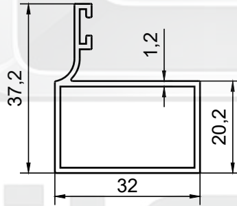
PROFİL NO : 136 AĞIRLIK : 0.411 Kg/m
