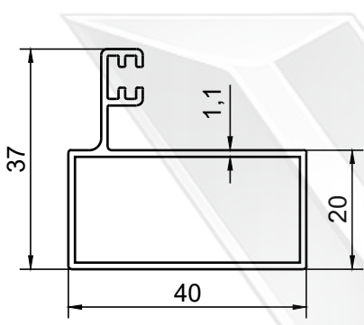
PROFİL NO : 323 AĞIRLIK : 0.453 Kg/m
