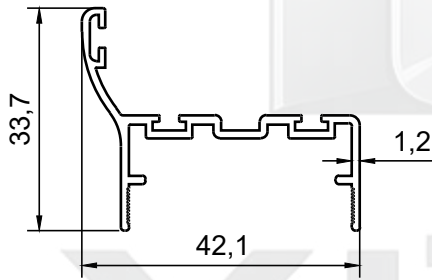
PROFİL NO : 1531 AĞIRLIK : 0.369 Kg/m
