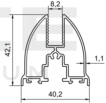
PROFİL NO : 2773 AĞIRLIK : 0.875 Kg/m
