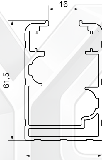
PROFİL NO : 1909 AĞIRLIK : 1.360 Kg/m
