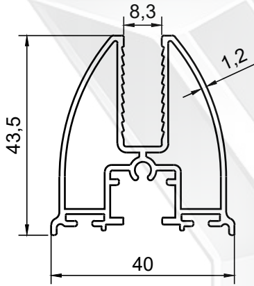
PROFİL NO : 2475 AĞIRLIK : 0.791 Kg/m
