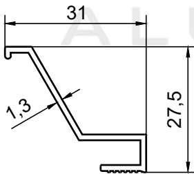
PROFİL NO : 2414 AĞIRLIK : 0.209 Kg/m
