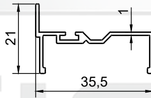
PROFİL NO : 1475 AĞIRLIK : 0.220 Kg/m
