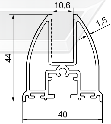
PROFİL NO : 1367 AĞIRLIK : 0.997 Kg/m
