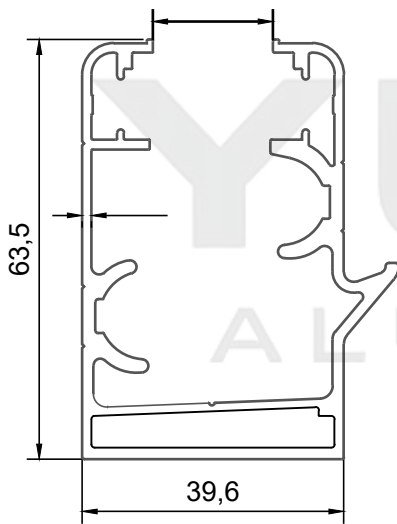
PROFİL NO : 321 AĞIRLIK : 1.309 Kg/m
