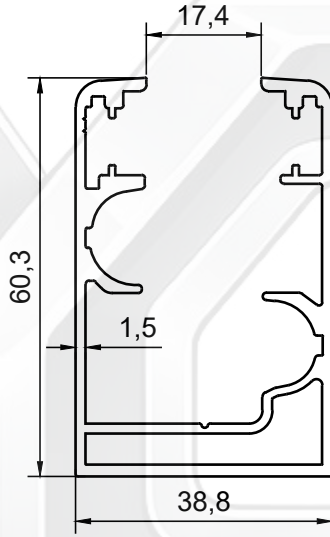
PROFİL NO : 2289 AĞIRLIK : 1.184 Kg/m
