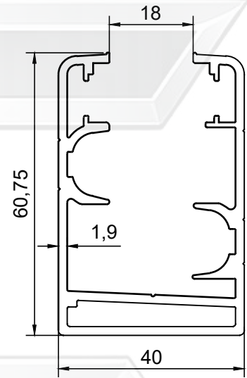
PROFİL NO : 133 AĞIRLIK : 1.366 Kg/m
