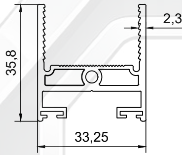
PROFİL NO : 1532 AĞIRLIK : 0.726 Kg/m
