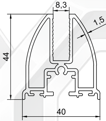
PROFİL NO : 132 AĞIRLIK : 0.997 Kg/m
