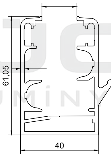
PROFİL NO : 1452 AĞIRLIK : 1.553 Kg/m
