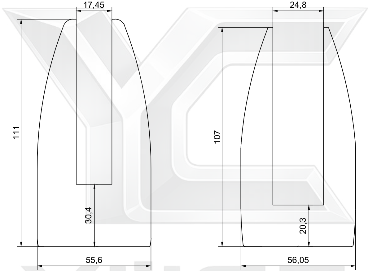
PROFİL NO : 2033 AĞIRLIK : 11.070 Kg/m
