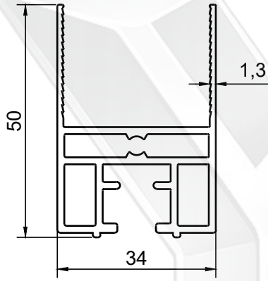
PROFİL NO : 1474 AĞIRLIK : 0.867 Kg/m
