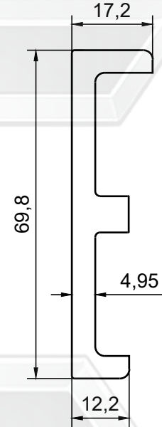
PROFİL NO : 2398 AĞIRLIK : 1.339 Kg/m
