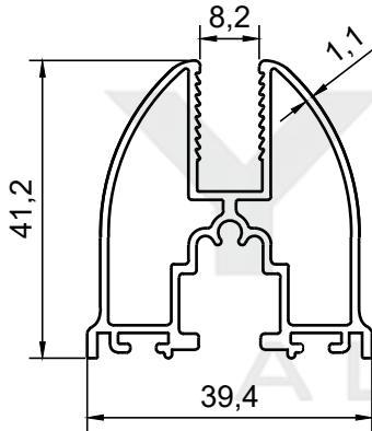
PROFİL NO : 2715 AĞIRLIK : 0.740 Kg/m
