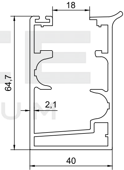
PROFİL NO : 1496 AĞIRLIK : 1.564 Kg/m
