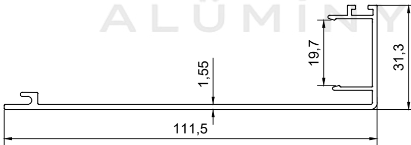
PROFİL NO : 2399 AĞIRLIK : 0.696 Kg/m
