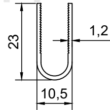
PROFİL NO : 1467 AĞIRLIK : 0.153 Kg/m
