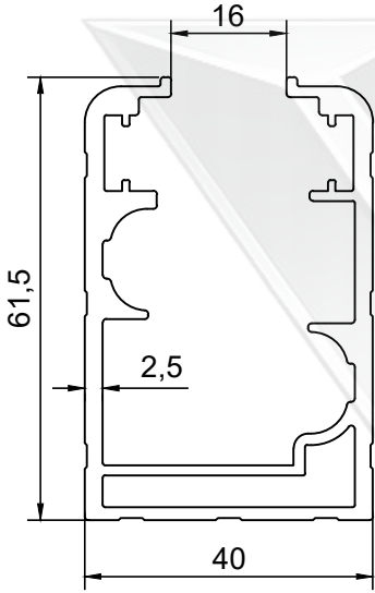
PROFİL NO : 320 AĞIRLIK : 1.474 Kg/m
