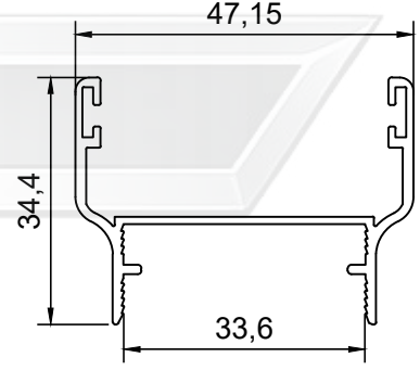
PROFİL NO : 1504 AĞIRLIK : 0.438 Kg/m
