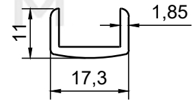
PROFİL NO : 2505 AĞIRLIK : 0.182 Kg/m
