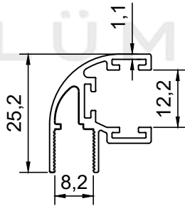
PROFİL NO : 341 AĞIRLIK : 0.311 Kg/m
