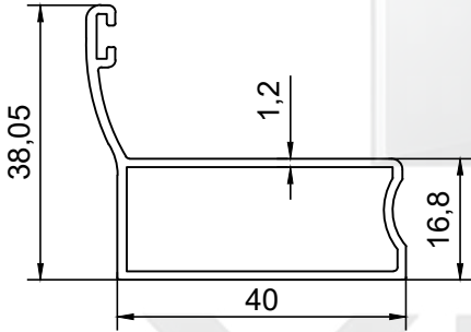
PROFİL NO : 1530 AĞIRLIK : 0.463 Kg/m
