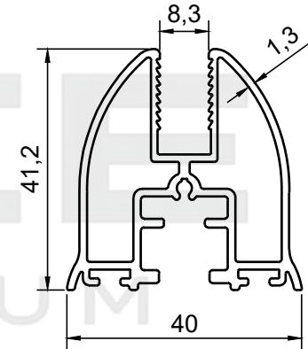
PROFİL NO : 1910 AĞIRLIK : 0.848 Kg/m
