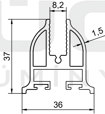
PROFİL NO : 131 AĞIRLIK : 0.875 Kg/m
