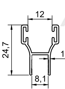
PROFİL NO : 1349 AĞIRLIK : 0.201 Kg/m
