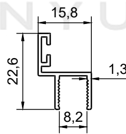
PROFİL NO : 326 AĞIRLIK : 0.165 Kg/m
