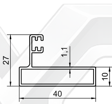
PROFİL NO : 349 AĞIRLIK : 0.393 Kg/m
