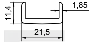
PROFİL NO : 2506 AĞIRLIK : 0.241 Kg/m
