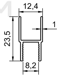
PROFİL NO : 325 AĞIRLIK : 0.164 Kg/m
