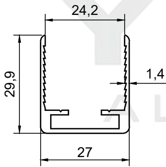
PROFİL NO : 2405 AĞIRLIK : 0.377 Kg/m
