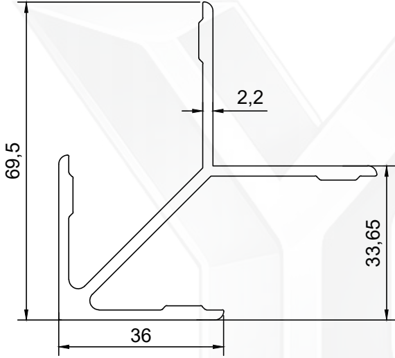
PROFİL NO : 330 AĞIRLIK : 1.238 Kg/m
