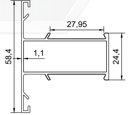
PROFİL NO : 237 AĞIRLIK : 0.580 Kg/m
