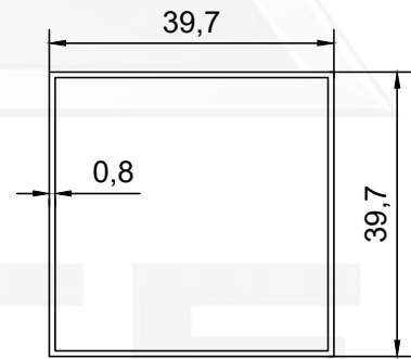
PROFİL NO : 304 AĞIRLIK : 0.337 Kg/m
