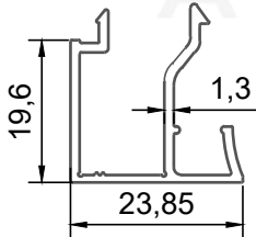
PROFİL NO : 2099 AĞIRLIK : 0.279 Kg/m
