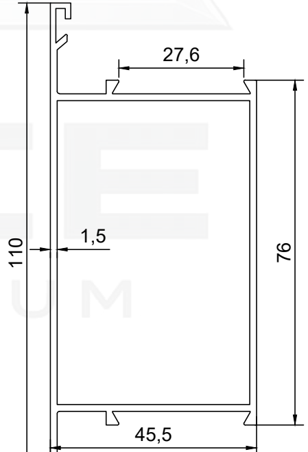
PROFİL NO : 224 AĞIRLIK : 1.190 Kg/m
