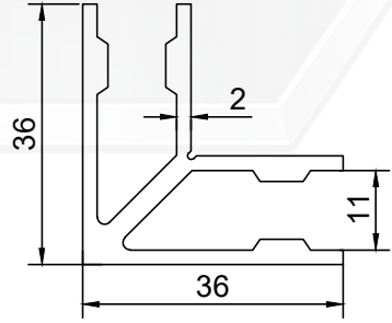
PROFİL NO : 2214 AĞIRLIK : 0.861 Kg/m
