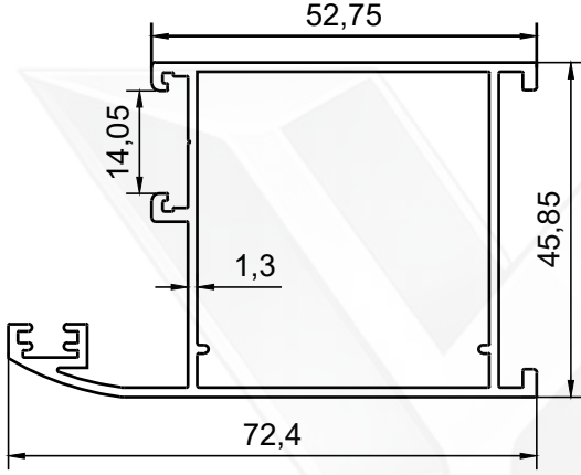
PROFİL NO : 2098 AĞIRLIK : 0.908 Kg/m
