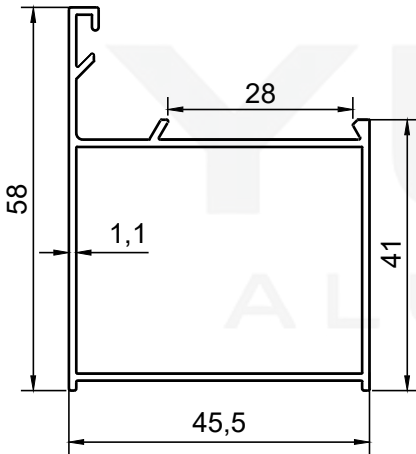
PROFİL NO : 337 AĞIRLIK : 0.599 Kg/m
