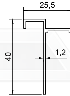
PROFİL NO : 2813 AĞIRLIK : 0.228 Kg/m
