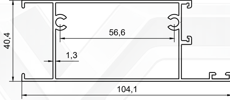
PROFİL NO : 2096 AĞIRLIK : 1.133 Kg/m
