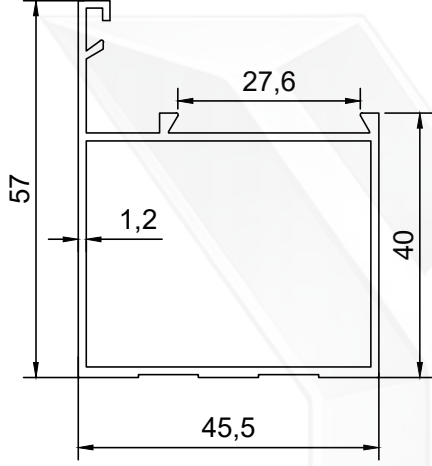
PROFİL NO : 220 AĞIRLIK : 0.674 Kg/m
