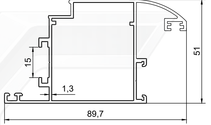
PROFİL NO : 2094 AĞIRLIK : 1.111 Kg/m
