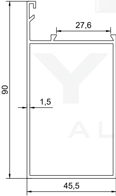
PROFİL NO : 223 AĞIRLIK : 1.052 Kg/m
