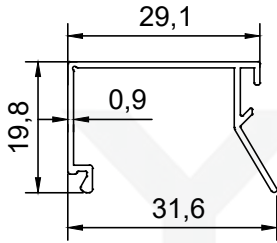
PROFİL NO : 227 AĞIRLIK : 0.190 Kg/m
