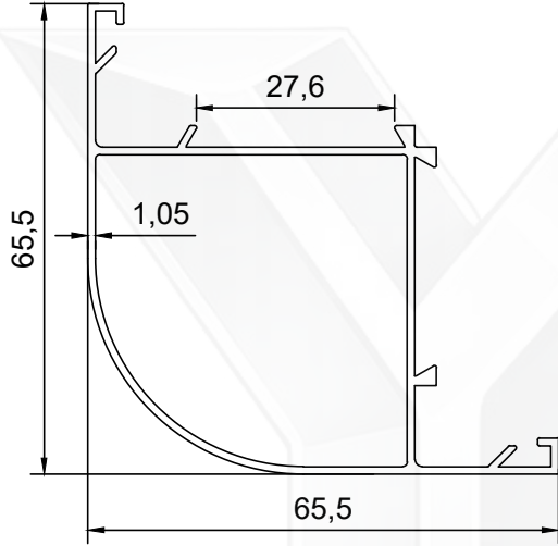
PROFİL NO : 1615 AĞIRLIK : 0.694 Kg/m
