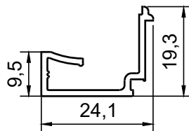
PROFİL NO : 2100 AĞIRLIK : 0.207 Kg/m
