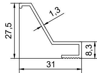
PROFİL NO : 2414 AĞIRLIK : 0.209 Kg/m
