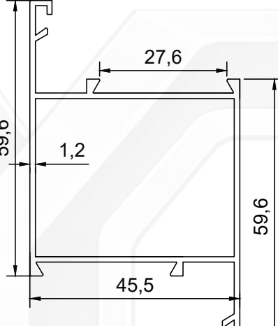
PROFİL NO : 222 AĞIRLIK : 0.772 Kg/m
