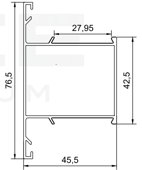
PROFİL NO : 338 AĞIRLIK : 0.704 Kg/m
