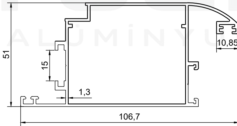
PROFİL NO : 2095 AĞIRLIK : 1.233 Kg/m
