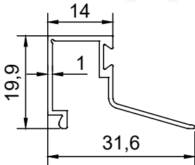
PROFİL NO : 228 AĞIRLIK : 0.201 Kg/m
