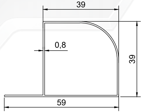
PROFİL NO : 306 AĞIRLIK : 0.362 Kg/m
