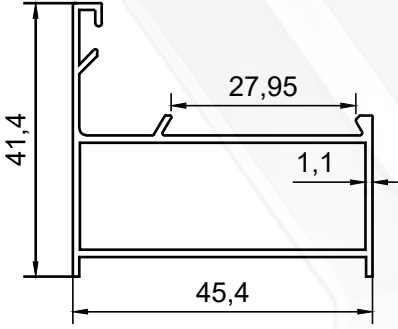
PROFİL NO : 239 AĞIRLIK : 0.490 Kg/m
