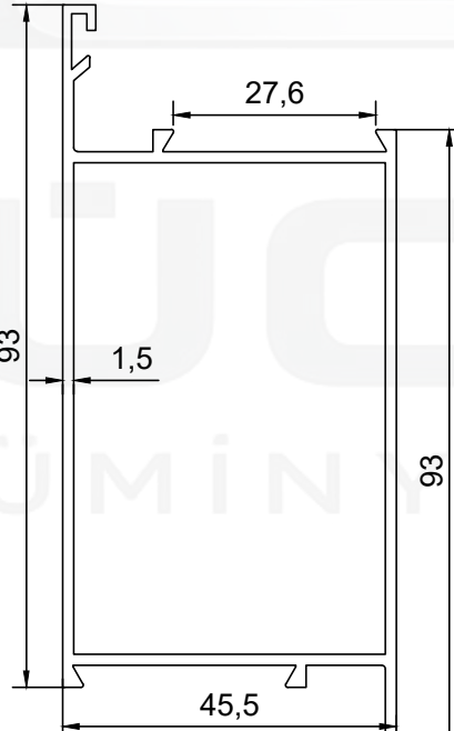
PROFİL NO : 225 AĞIRLIK : 1.190 Kg/m
