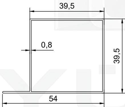
PROFİL NO : 305 AĞIRLIK : 0.371 Kg/m
