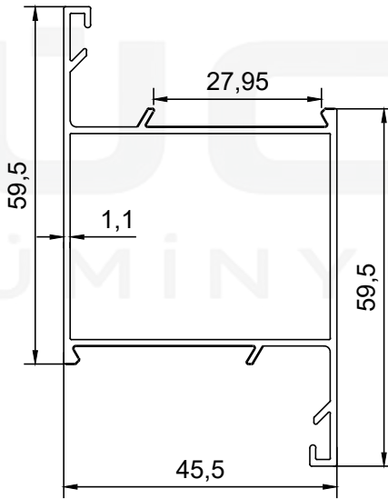
PROFİL NO : 339 AĞIRLIK : 0.704 Kg/m
