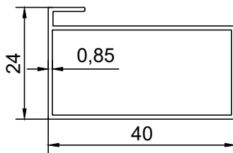
PROFİL NO : 307 AĞIRLIK : 0.295 Kg/m
