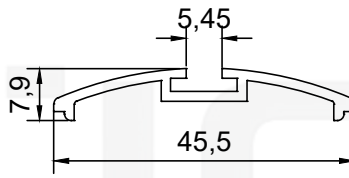
PROFİL NO : 2811 AĞIRLIK : 0.257 Kg/m
