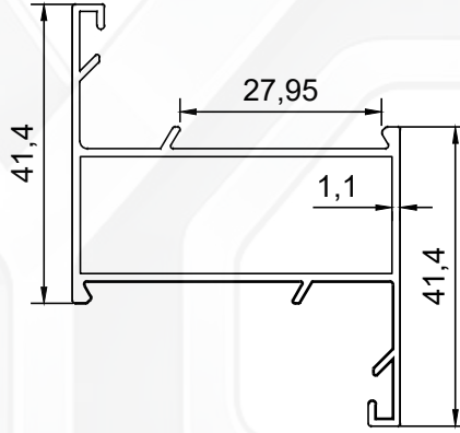
PROFİL NO : 238 AĞIRLIK : 0.580 Kg/m
