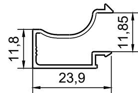
PROFİL NO : 2531 AĞIRLIK : 0.187 Kg/m
