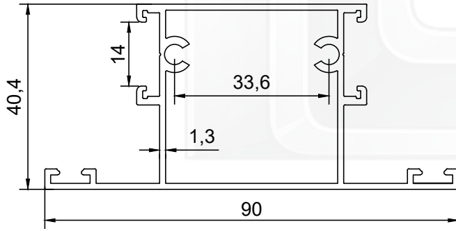
PROFİL NO : 2093 AĞIRLIK : 1.015 Kg/m
