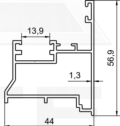
PROFİL NO : 2097 AĞIRLIK : 0.761 Kg/m
