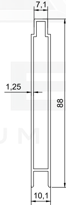
PROFİL NO : 226 AĞIRLIK : 0.646 Kg/m
