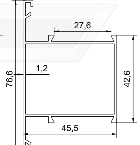
PROFİL NO : 221 AĞIRLIK : 0.770 Kg/m
