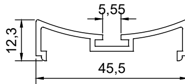
PROFİL NO : 2812 AĞIRLIK : 0.336 Kg/m
