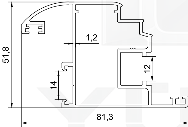
PROFİL NO : 2092 AĞIRLIK : 1.149 Kg/m
