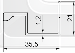
PROFİL NO : 1430 AĞIRLIK : 0.287 Kg/m
