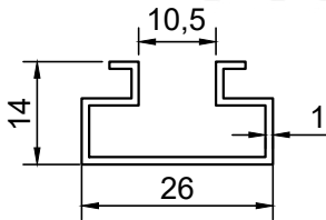
PROFİL NO : 1429 AĞIRLIK : 0.195 Kg/m
