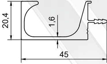
PROFİL NO : 1435 AĞIRLIK : 0.566 Kg/m
