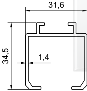
PROFİL NO : 1434 AĞIRLIK : 0.445 Kg/m
