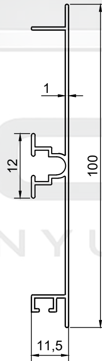
PROFİL NO : 1437 AĞIRLIK : 0.463 Kg/m
