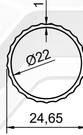
PROFİL NO : 1512 AĞIRLIK : 0.217 Kg/m
