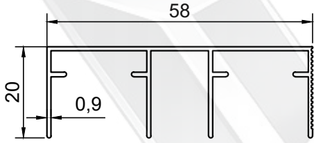
PROFİL NO : 1439 AĞIRLIK : 0.354 Kg/m
