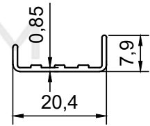
PROFİL NO : 1426 AĞIRLIK : 0.087 Kg/m
