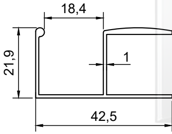
PROFİL NO : 1431 AĞIRLIK : 0.336 Kg/m
