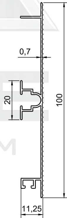
PROFİL NO : 1428 AĞIRLIK : 0.385 Kg/m
