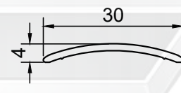
PROFİL NO : 1289 AĞIRLIK : 0.122 Kg/m
