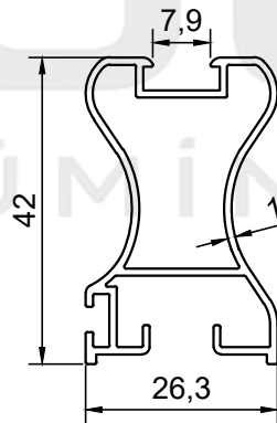
PROFİL NO : 1441 AĞIRLIK : 0.458 Kg/m
