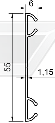
PROFİL NO : 1436 AĞIRLIK : 0.238 Kg/m
