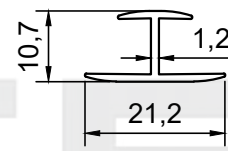
PROFİL NO : 1528 AĞIRLIK : 0.117 Kg/m
