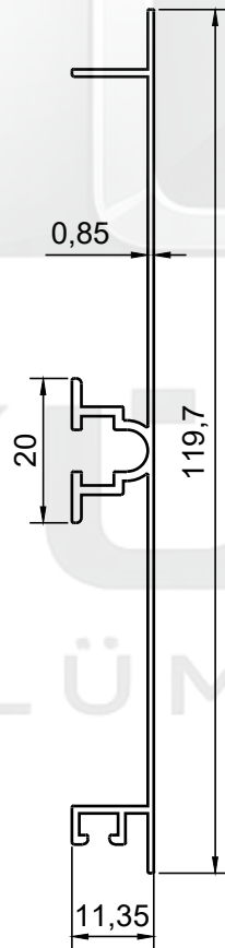
PROFİL NO : 1757 AĞIRLIK : 0.154 Kg/m
