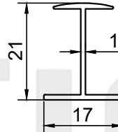
PROFİL NO : 1433 AĞIRLIK : 0.138 Kg/m
