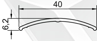
PROFİL NO : 1319 AĞIRLIK : 0.168 Kg/m
