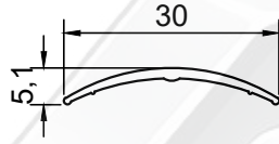
PROFİL NO : 1318 AĞIRLIK : 0.108 Kg/m
