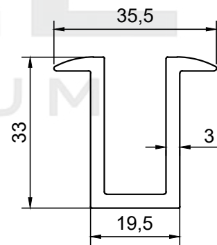
PROFİL NO : 1361 AĞIRLIK : 0.743 Kg/m
