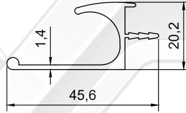
PROFİL NO : 1427 AĞIRLIK : 0.430 Kg/m
