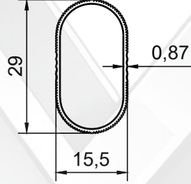
PROFİL NO : 1757 AĞIRLIK : 0.154 Kg/m
