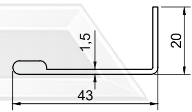
PROFİL NO : 1519 AĞIRLIK : 0.309 Kg/m
