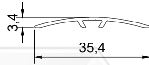
PROFİL NO : 1513 AĞIRLIK : 0.112 Kg/m
