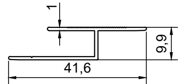
PROFİL NO : 1521 AĞIRLIK : 0.171 Kg/m
