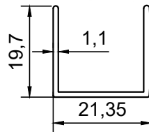
PROFİL NO : 1432 AĞIRLIK : 0.195 Kg/m
