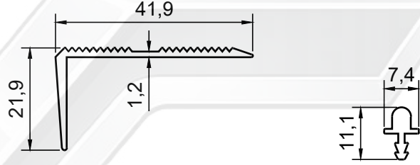
PROFİL NO : 1515 AĞIRLIK : 0.261 Kg/m
