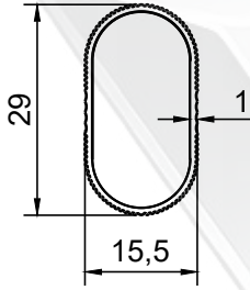
PROFİL NO : 1425 AĞIRLIK : 0.176 Kg/m
