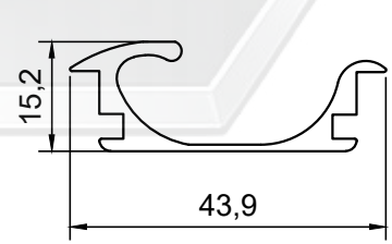
PROFİL NO : 1514 AĞIRLIK : 0.404 Kg/m
