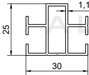
PROFİL NO : 1593 AĞIRLIK : 0.385 Kg/m
