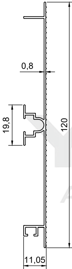
PROFİL NO : 1425 AĞIRLIK : 0.176 Kg/m
