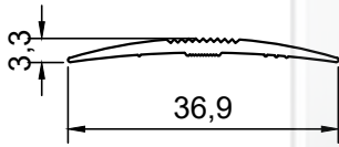
PROFİL NO : 1274 AĞIRLIK : 0.152 Kg/m
