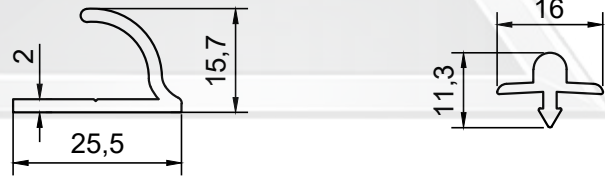
PROFİL NO : 1360 AĞIRLIK : 0.249 Kg/m
