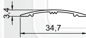
PROFİL NO : 1438 AĞIRLIK : 0.115 Kg/m
