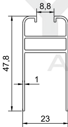
PROFİL NO : 1537 AĞIRLIK : 0.428 Kg/m
