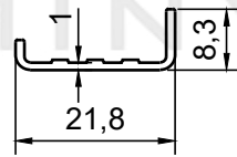
PROFİL NO : 1518 AĞIRLIK : 0.095 Kg/m
