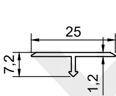
PROFİL NO : 1290 AĞIRLIK : 0.099 Kg/m
