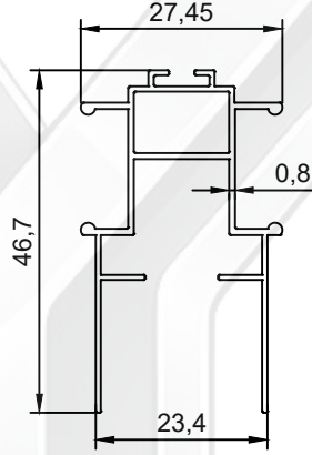
PROFİL NO : 2111 AĞIRLIK : 0.344 Kg/m
