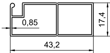
PROFİL NO : 1324 AĞIRLIK : 0.328 Kg/m
