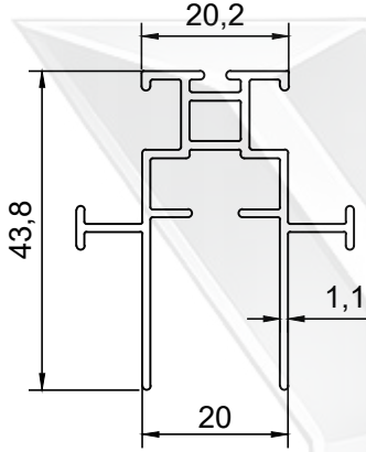
PROFİL NO : 297 AĞIRLIK : 0.520 Kg/m
