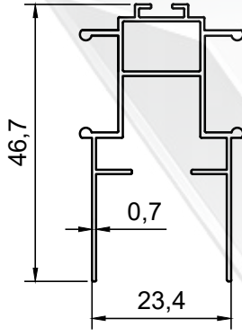
PROFİL NO : 2677 AĞIRLIK : 0.344 Kg/m
