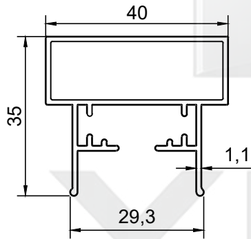
PROFİL NO : 295 AĞIRLIK : 0.526 Kg/m
