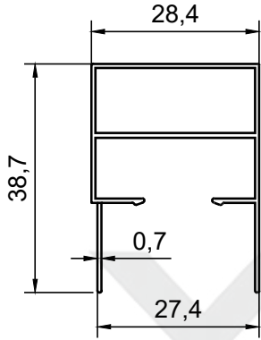
PROFİL NO : 2676 AĞIRLIK : 0.287 Kg/m
