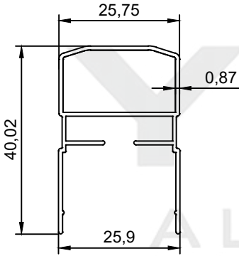
PROFİL NO : 2051 AĞIRLIK : 0.322 Kg/m
