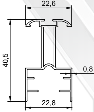
PROFİL NO : 2052 AĞIRLIK : 0.325 Kg/m
