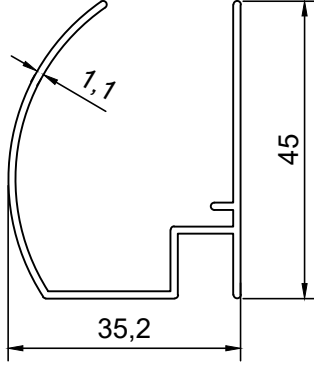
PROFİL NO : 1344 AĞIRLIK : 0.407 Kg/m
