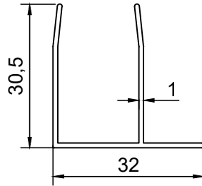
PROFİL NO : 1345 AĞIRLIK : 0.247 Kg/m
