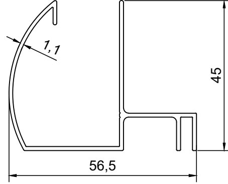
PROFİL NO : 2069 AĞIRLIK : 0.542 Kg/m
