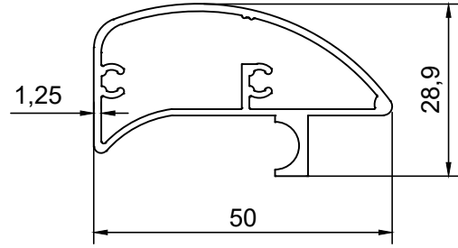
PROFİL NO : 1346 AĞIRLIK : 0.569 Kg/m
