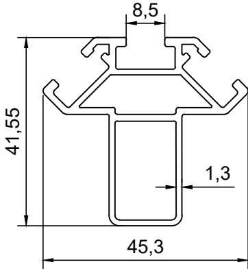
PROFİL NO : 1211 AĞIRLIK : 0.734 Kg/m
