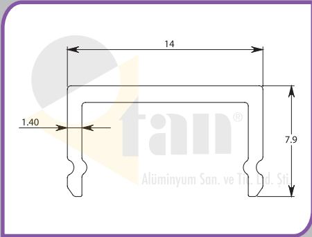
Profil 10-0013 Profile 10-0013 مقطع 10-0013
