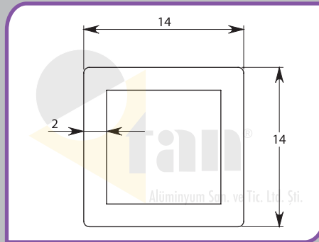
Profil 10-0005 Profile 10-0005 مقطع 10-0005
