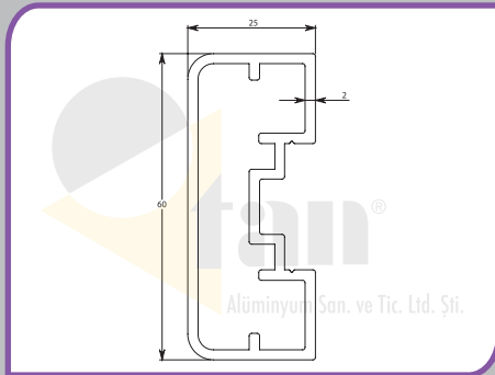
Profil 10-0004 Profile 10-0004 مقطع 10-0004
