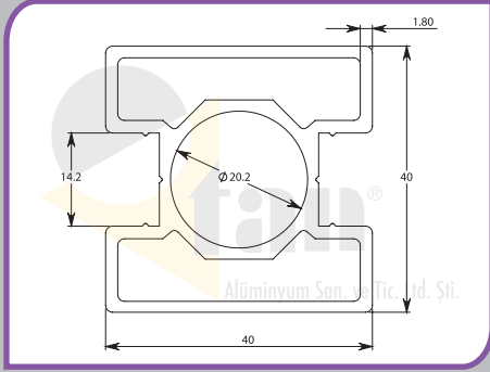
Profil 10-0001 Profile 10-0001 مقطع 10-0001
