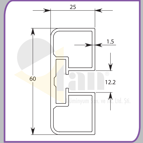
Profil 10-0012 Profile 10-0012 مقطع 10-0012
