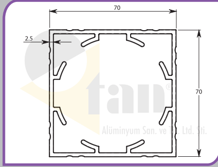
Profil 10-0002 Profile 10-0002 مقطع 10-0002
