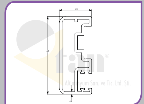
Profil 10-0009 Profile 10-0009 مقطع 10-0009
