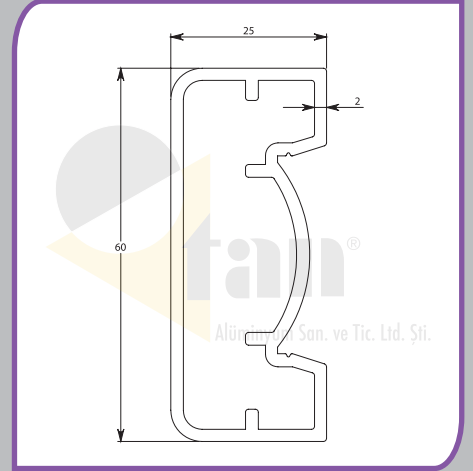
Profil 10-0003 Profile 10-0003 مقطع 10-0003
