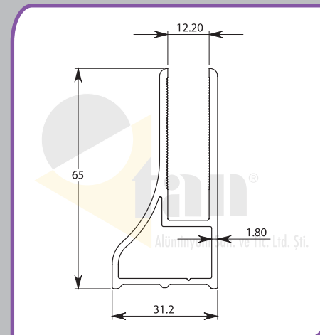
Profil 10-0017 Profile 10-0017 مقطع 10-0017
