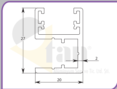
Profil 10-0007 Profile 10-0007 مقطع 10-0007
