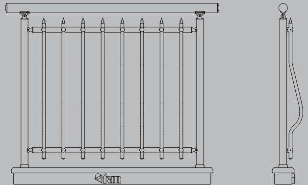
Uygulama 10 Teknik Resim Application 10 Technical Drawing تطبيق 10 رسم فني
