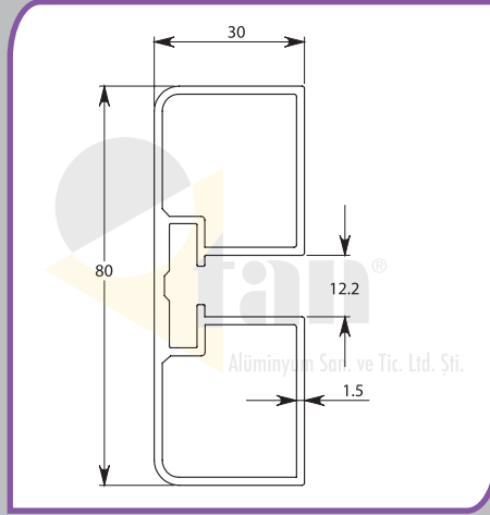
Profil 10-0011 Profile 10-0011 مقطع 10-0011
