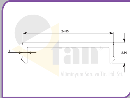
Profil 10-0014 Profile 10-0014 مقطع 10-0014
