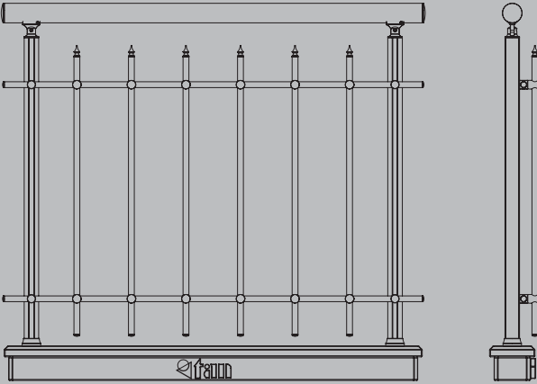
Uygulama 1 Teknik Resim Application 1 Technical Drawing تطبيق 1 رسم فني
