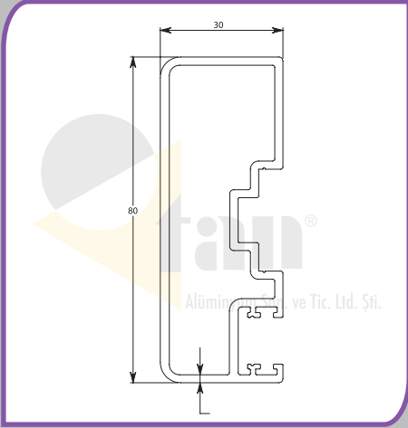
Profil 10-0010 Profile 10-0010 مقطع 10-0010
