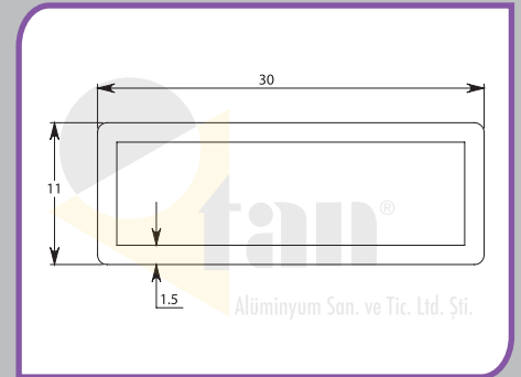
Profil 10-0006 Profile 10-0006 مقطع 10-0006
