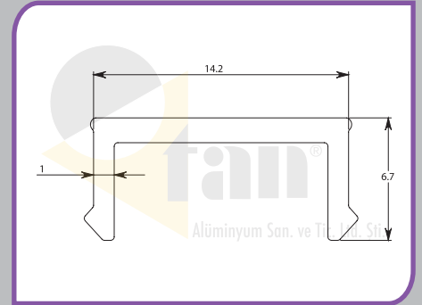
Profil 10-0015 Profile 10-0015 مقطع 10-0015
