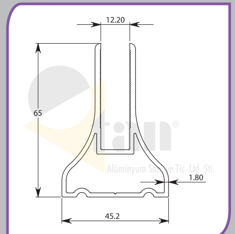
Profil 10-0018 Profile 10-0018 مقطع 10-0018
