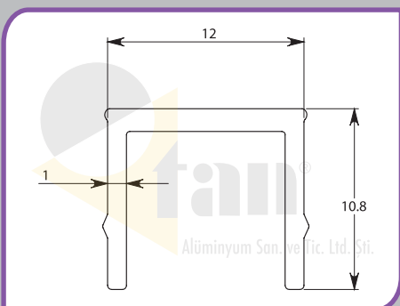
Profil 10-0016 Profile 10-0016 مقطع 10-0016
