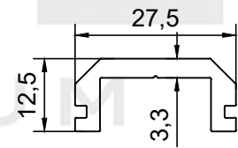
PROFİL NO : 275 AĞIRLIK : 0.384 Kg/m
