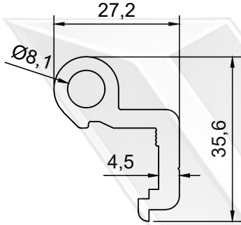
PROFİL NO : 095 AĞIRLIK : 0.737 Kg/m
