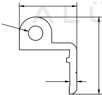
PROFİL NO : 1568 AĞIRLIK : 0.818 Kg/m
