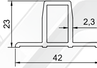
PROFİL NO : 291 AĞIRLIK : 0.504 Kg/m
