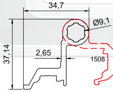
PROFİL NO : 1509 AĞIRLIK : 0.626 Kg/m
