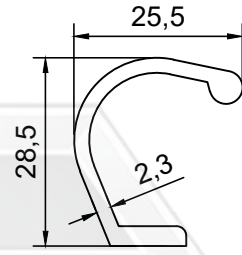
PROFİL NO : 367 AĞIRLIK : 0.404 Kg/m
