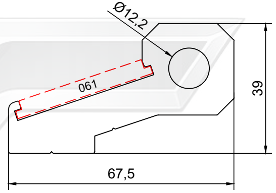
PROFİL NO : 090 AĞIRLIK : 3.062 Kg/m
