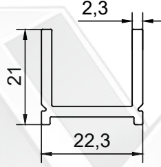
PROFİL NO : 1511 AĞIRLIK : 0.363 Kg/m
