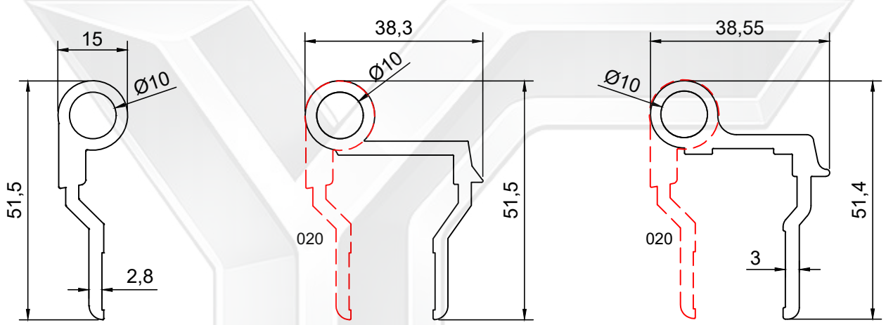
PROFİL NO : 020 AĞIRLIK : 0.659 Kg/m
