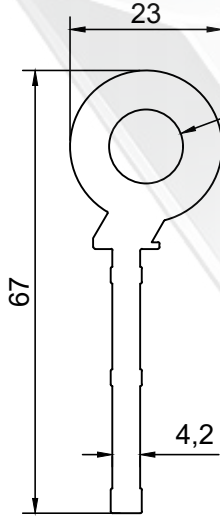
PROFİL NO : 052A AĞIRLIK : 1.438 Kg/m
