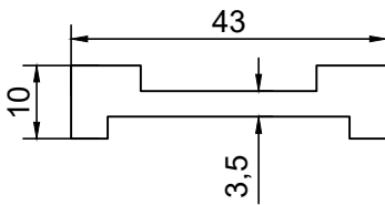
PROFİL NO : 059 AĞIRLIK : 0.669 Kg/m
