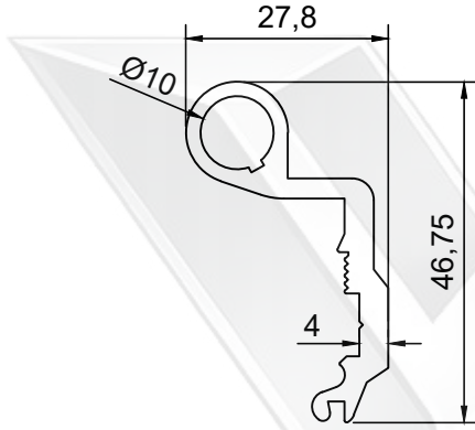
PROFİL NO : 102 AĞIRLIK : 0.699 Kg/m
