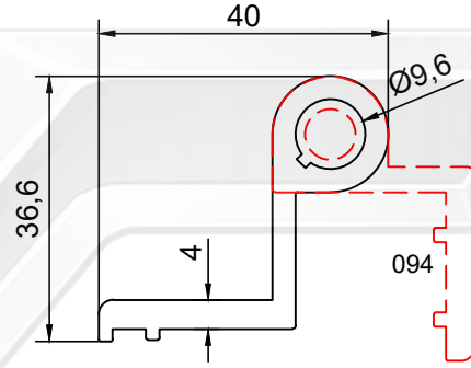
PROFİL NO : 093 AĞIRLIK : 0.820 Kg/m
