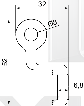
PROFİL NO : 270 AĞIRLIK : 1.359 Kg/m
