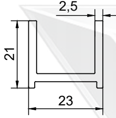
PROFİL NO : 1507 AĞIRLIK : 0.400 Kg/m
