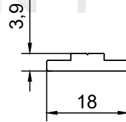
PROFİL NO : 064 AĞIRLIK : 0.146 Kg/m
