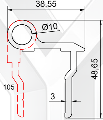
PROFİL NO : 085 AĞIRLIK : 0.781 Kg/m
