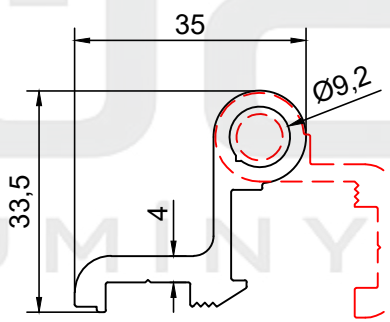
PROFİL NO : 099 AĞIRLIK : 0.717 Kg/m
