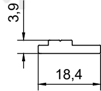
PROFİL NO : 063 AĞIRLIK : 0.148 Kg/m
