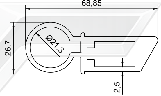
PROFİL NO : 292 AĞIRLIK : 1.441 Kg/m
