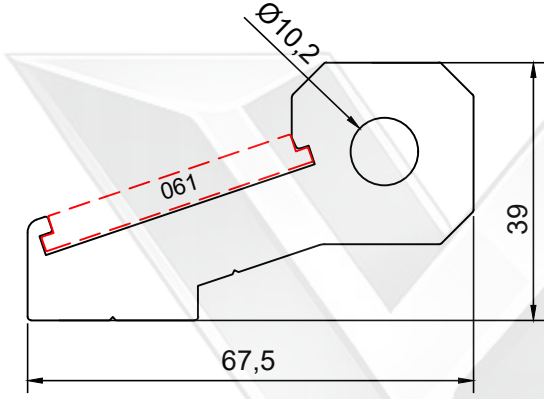
PROFİL NO : 089 AĞIRLIK : 3.157 Kg/m
