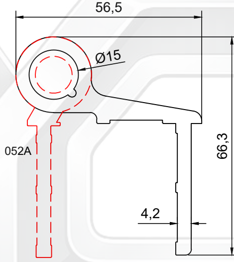
PROFİL NO : 053A AĞIRLIK : 1.695 Kg/m
