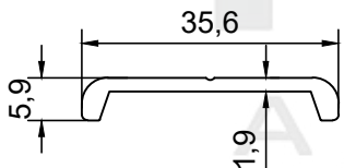
PROFİL NO : 1911 AĞIRLIK : 0.233 Kg/m
