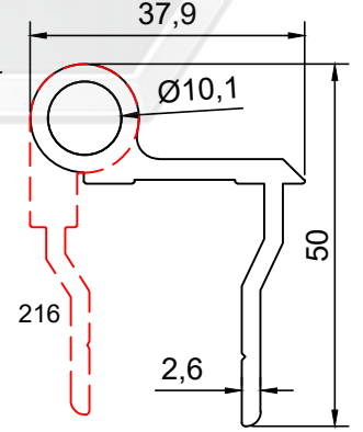
PROFİL NO : 211 AĞIRLIK : 0.745 Kg/m
