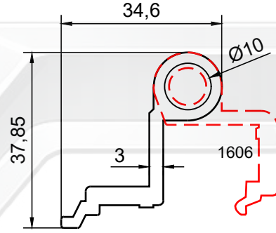
PROFİL NO : 1605 AĞIRLIK : 0.646 Kg/m
