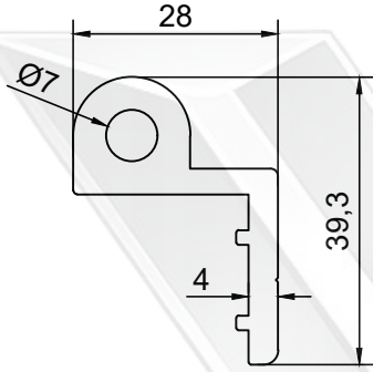
PROFİL NO : 094 AĞIRLIK : 0.897 Kg/m
