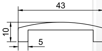
PROFİL NO : 214 AĞIRLIK : 0.512 Kg/m
