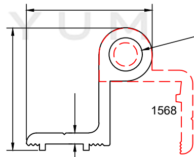
PROFİL NO : 166 AĞIRLIK : 0.751 Kg/m
