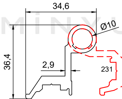
PROFİL NO : 232 AĞIRLIK : 0.618 Kg/m
