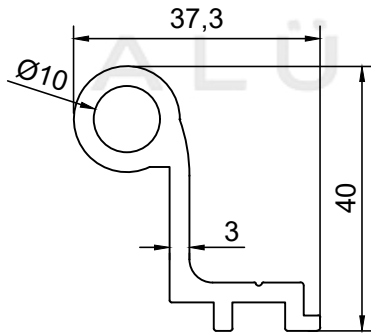
PROFİL NO : 1354 AĞIRLIK : 0.768 Kg/m
