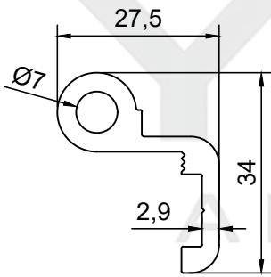
PROFİL NO : 100 AĞIRLIK : 0.629 Kg/m
