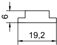
PROFİL NO : 179 AĞIRLIK : 0.242 Kg/m
