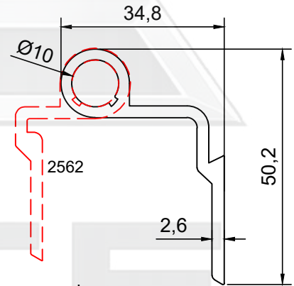
PROFİL NO : 2561 AĞIRLIK : 0.649 Kg/m
