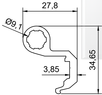
PROFİL NO : 1508 AĞIRLIK : 0.575 Kg/m
