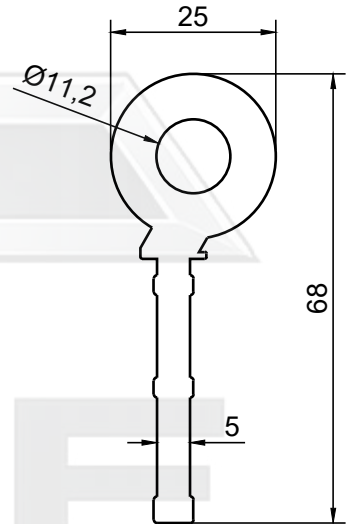
PROFİL NO : 052 AĞIRLIK : 1.718 Kg/m
