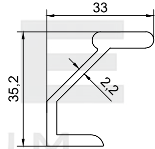
PROFİL NO : 280 AĞIRLIK : 0.626 Kg/m
