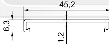
PROFİL NO : 1330 AĞIRLIK : 0.195 Kg/m
