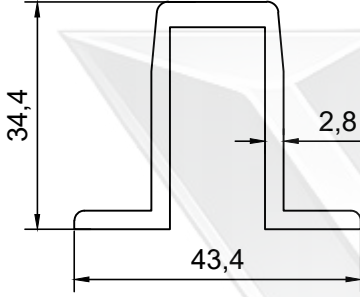
PROFİL NO : 1362 AĞIRLIK : 0.815 Kg/m
