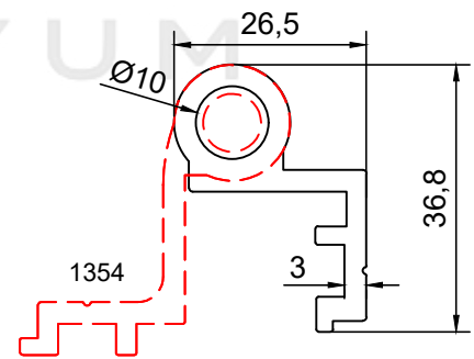
PROFİL NO : 1355 AĞIRLIK : 0.801 Kg/m
