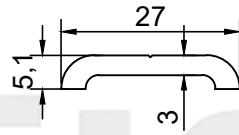
PROFİL NO : 034 AĞIRLIK : 0.237 Kg/m
