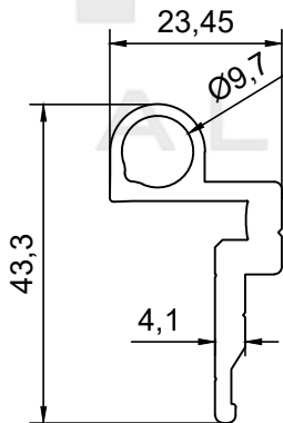
PROFİL NO : 097 AĞIRLIK : 0.644 Kg/m
