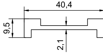
PROFİL NO : 106 AĞIRLIK : 0.462 Kg/m
