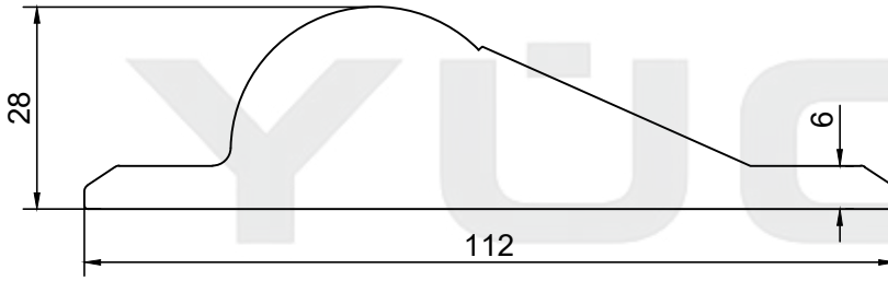
PROFİL NO : 047 AĞIRLIK : 4.377 Kg/m
