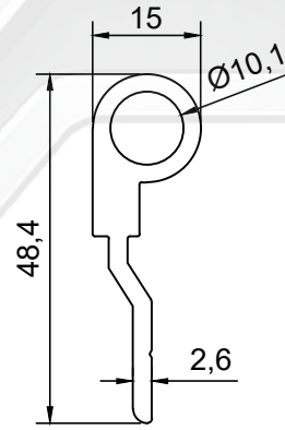
PROFİL NO : 216 AĞIRLIK : 0.721 Kg/m
