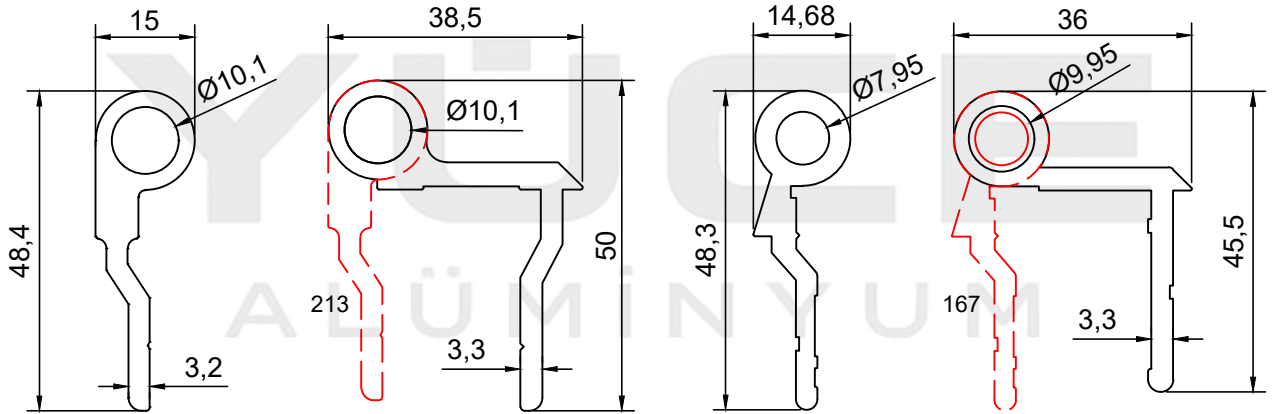
PROFİL NO : 213 AĞIRLIK : 0.659 Kg/m
