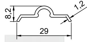
PROFİL NO : 1342 AĞIRLIK : 0.138 Kg/m
