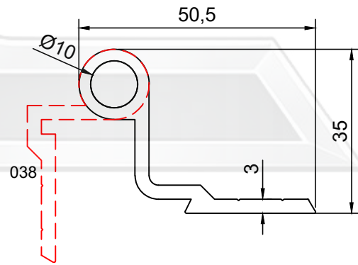
PROFİL NO : 037 AĞIRLIK : 0.743 Kg/m
