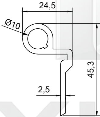
PROFİL NO : 2562 AĞIRLIK : 0.595 Kg/m
