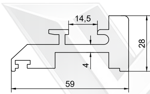
PROFİL NO : 110 AĞIRLIK : 1.753 Kg/m
