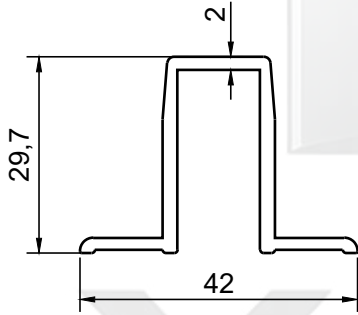
PROFİL NO : 293 AĞIRLIK : 0.531 Kg/m
