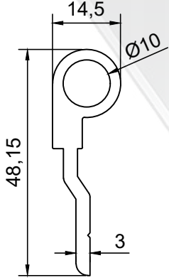
PROFİL NO : 105 AĞIRLIK : 0.602 Kg/m
