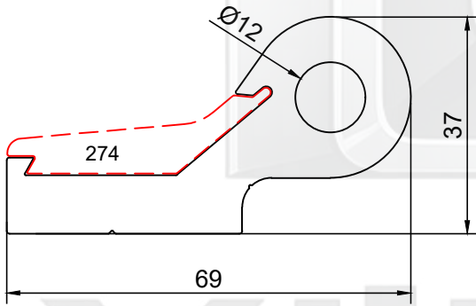
PROFİL NO : 273 AĞIRLIK : 2.721 Kg/m
