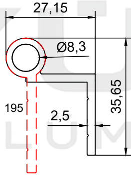
PROFİL NO : 196 AĞIRLIK : 0.447 Kg/m
