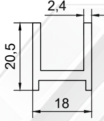
PROFİL NO : 1363 AĞIRLIK : 0.364 Kg/m
