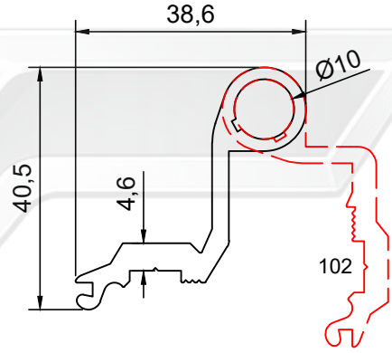
PROFİL NO : 101 AĞIRLIK : 0.697 Kg/m
