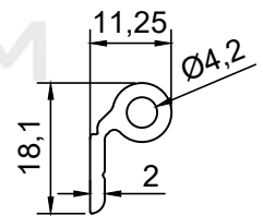
PROFİL NO : 1225 AĞIRLIK : 0.178 Kg/m
