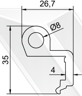
PROFİL NO : 1606 AĞIRLIK : 0.710 Kg/m
