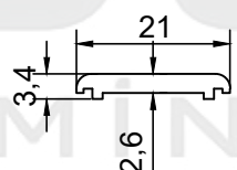
PROFİL NO : 1914 AĞIRLIK : 0.146 Kg/m
