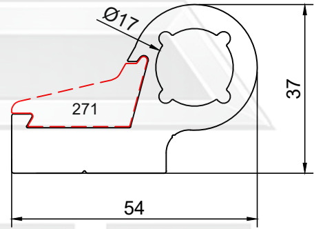
PROFİL NO : 272 AĞIRLIK : 1.947 Kg/m
