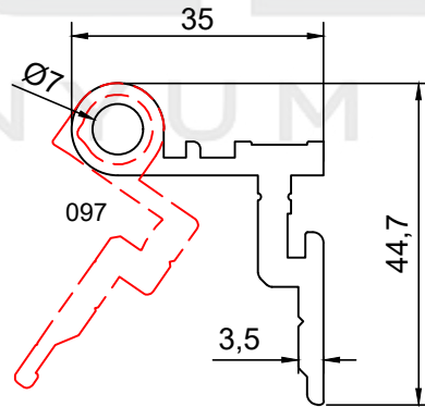
PROFİL NO : 098 AĞIRLIK : 0.886 Kg/m
