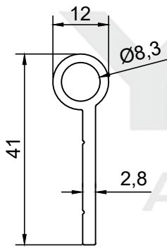
PROFİL NO : 195 AĞIRLIK : 0.382 Kg/m
