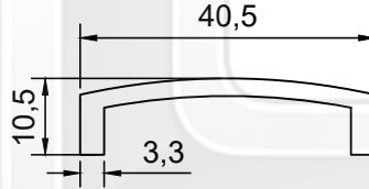
PROFİL NO : 107 AĞIRLIK : 0.376 Kg/m
