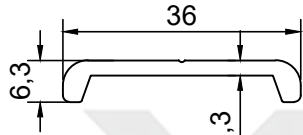
PROFİL NO : 149 AĞIRLIK : 0.282 Kg/m
