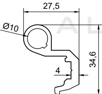
PROFİL NO : 231 AĞIRLIK : 0.588 Kg/m
