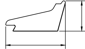
PROFİL NO : 271 AĞIRLIK : 0.631 Kg/m
