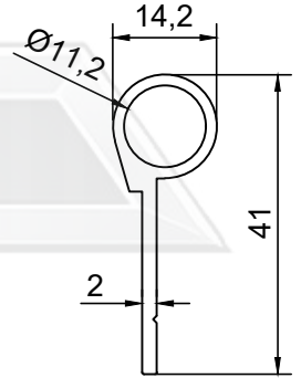
PROFİL NO : 103 AĞIRLIK : 0.331 Kg/m
