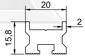
PROFİL NO : 062 AĞIRLIK : 0.529 Kg/m
