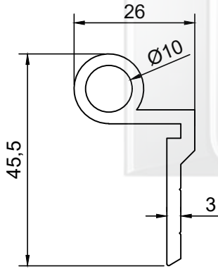
PROFİL NO : 038 AĞIRLIK : 0.659 Kg/m
