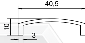
PROFİL NO : 343 AĞIRLIK : 0.291 Kg/m
