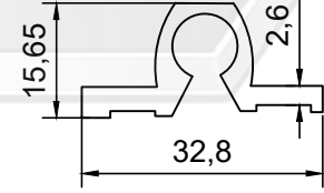
PROFİL NO : 1333 AĞIRLIK : 0.418 Kg/m
