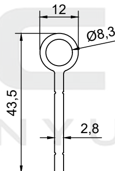
PROFİL NO : 194 AĞIRLIK : 0.398 Kg/m
