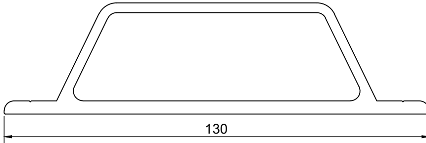
PROFİL NO : 280 AĞIRLIK : 0.626 Kg/m
