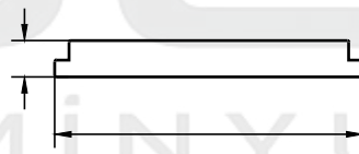
PROFİL NO : 061 AĞIRLIK : 0.549 Kg/m
