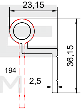
PROFİL NO : 193 AĞIRLIK : 0.425 Kg/m
