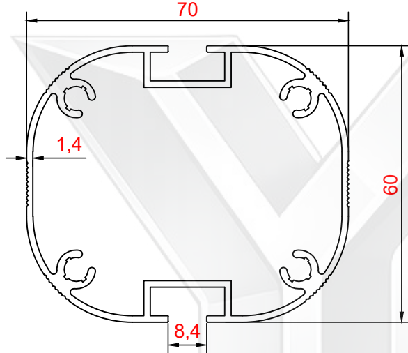
PROFİL NO : 397 AĞIRLIK : 1.309 Kg/m
