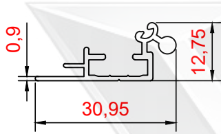
PROFİL NO : 1202 AĞIRLIK : 0.203 Kg/m
