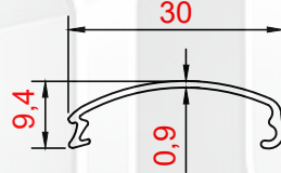
PROFİL NO : 1207 AĞIRLIK : 0.114 Kg/m
