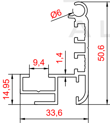
PROFİL NO : 1212 AĞIRLIK : 0.644 Kg/m
