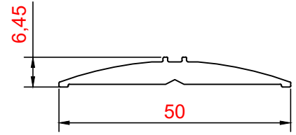
PROFİL NO : 1223 AĞIRLIK : 0.477 Kg/m
