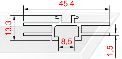
PROFİL NO : 1219 AĞIRLIK : 0.424 Kg/m
