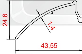
PROFİL NO : 1216 AĞIRLIK : 0.238 Kg/m
