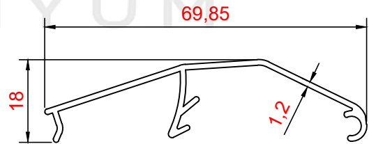
PROFİL NO : 1215 AĞIRLIK : 0.371 Kg/m
