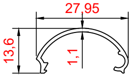
PROFİL NO : 1206 AĞIRLIK : 0.140 Kg/m
