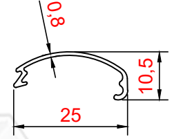
PROFİL NO : 1209 AĞIRLIK : 0.091 Kg/m
