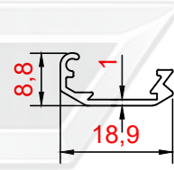
PROFİL NO : 1205 AĞIRLIK : 0.103 Kg/m
