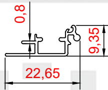
PROFİL NO : 1224 AĞIRLIK : 0.109 Kg/m
