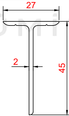
PROFİL NO : 1218 AĞIRLIK : 0.374 Kg/m
