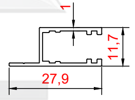
PROFİL NO : 1309 AĞIRLIK : 0.179 Kg/m
