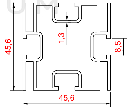
PROFİL NO : 1220 AĞIRLIK : 1.160 Kg/m
