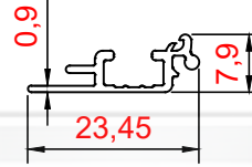
PROFİL NO : 1208 AĞIRLIK : 0.121 Kg/m
