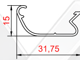
PROFİL NO : 1203 AĞIRLIK : 0.163 Kg/m
