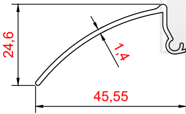
PROFİL NO : 1217 AĞIRLIK : 0.240 Kg/m
