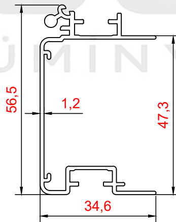
PROFİL NO : 1222 AĞIRLIK : 0.558 Kg/m
