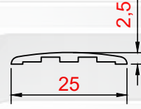
PROFİL NO : 1204 AĞIRLIK : 0.092 Kg/m
