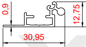
PROFİL NO : 1213 AĞIRLIK : 0.195 Kg/m
